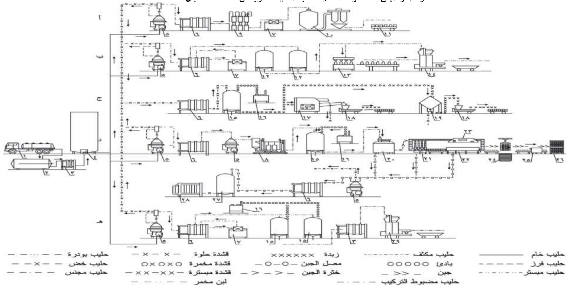
رسم توضيحي 4: خطوط الانتاج حسب المنتج المطلوب من مشتقات الألبان
